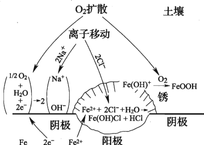
图 1 氧浓差电池的腐蚀模型
