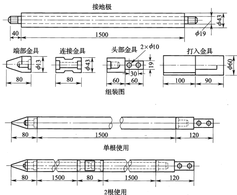
图 2 锌接地极结构图
